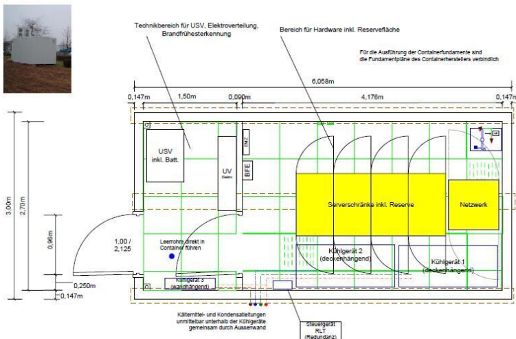
Grundriss, Klimatechnik und Doppelboden
